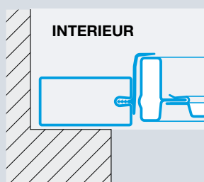
Type de porte N 80 Montage derrière le jour
