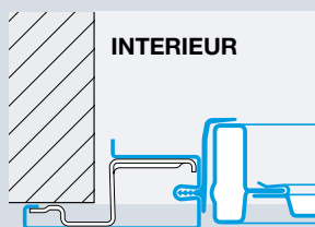
Type de porte F 80 Montage devant le jour
