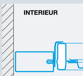
Type de porte N 80 Montage dans le jour
