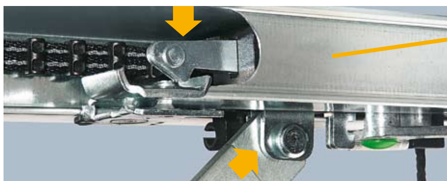
Le verrouillage de la porte dans le rail d'entraînement – un brevet Hörmann
